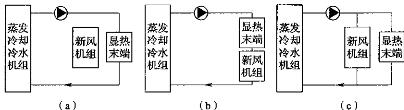
图 4 蒸发冷却水系统流程
