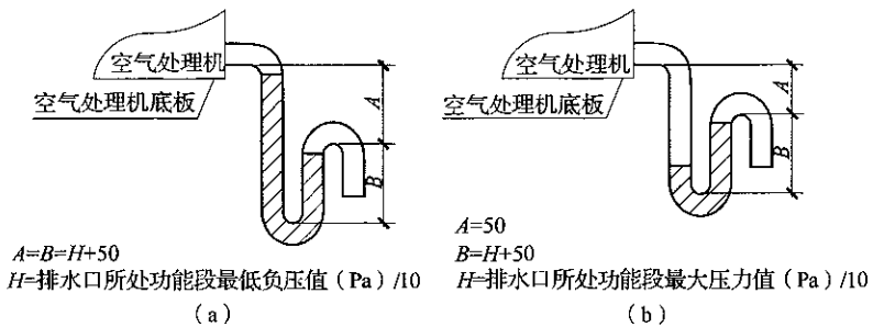
图 1 排水水封
